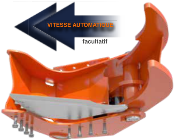
lame facilement remplaçable
